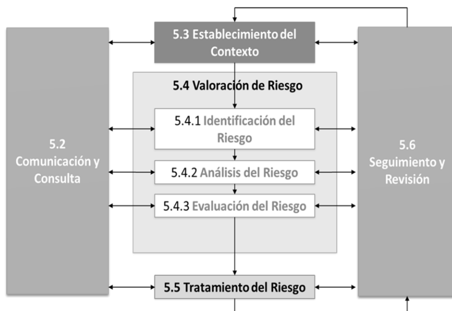
Ilustración 6. Análisis de Riesgos BCP
